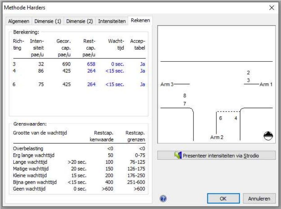
Kruispunt N50 met Kuurnsesteenweg (geplande situatie) - scenario ontsl. via N50
